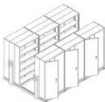
CPT-305 (3 แถว) 2540(L) x 3660(W) x 2250(H) mm.
