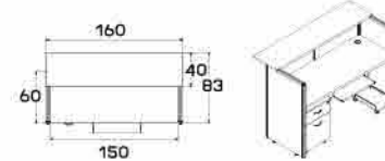
PREMIER SET 3 ขนาดรวม = 160 w x 83 d x 110 h cm.
