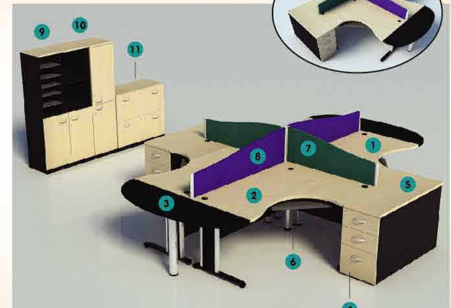
ขนาดรวมเฉพาะชุดโต๊ะ- 390 x 324 x 115 cm.
